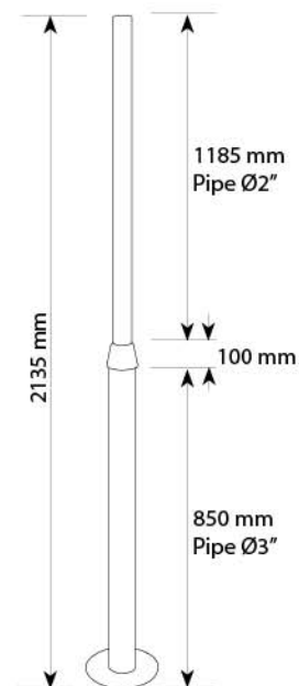
Product Code : 203 Pole Material : MS Base Dia : Ø225 mm
